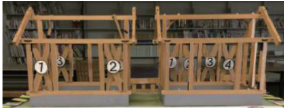
筋かいバランス模型
